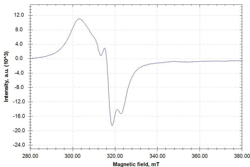
3-rasm. Apis Mellifera xitozaning \text{Cu}^{2+} metalli bilan kompleksi EPR-spektri
