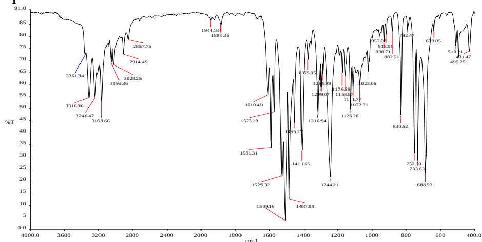
Рисунок 1. ИК-спектр бензоилгидразона 1-(3-фурила)-4,4,4-трифторбутандиона-1,3 ( H_2L^1 )
