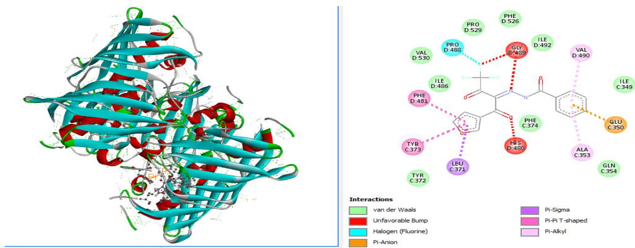
Рис.3. Результаты молекулярного докинга молекулы H_2L^1
