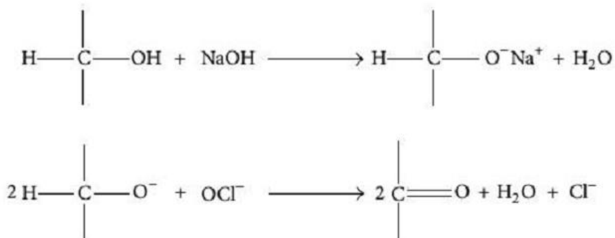
Схема 2 Окисление крахмала образованной гипохлоритом в щелочной среде
