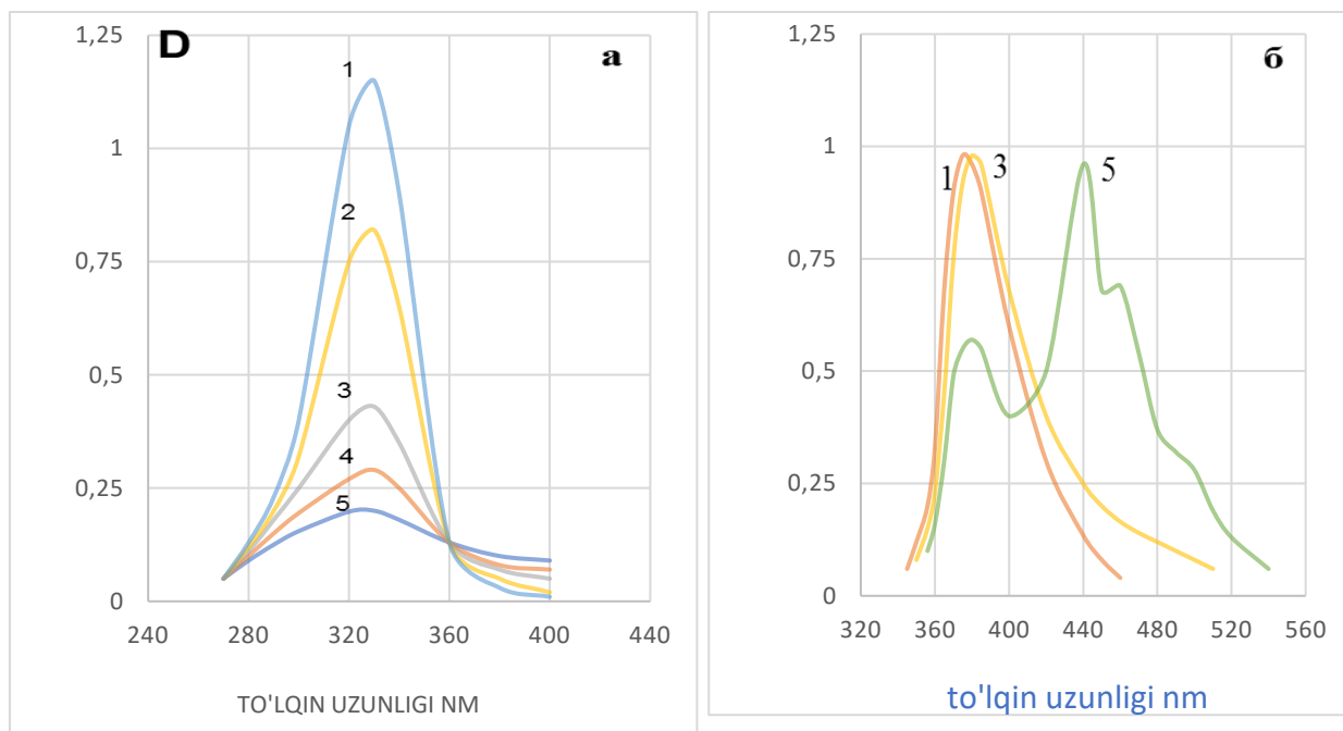
1-rasm. Doimiy dioksan-suv ikkilik aralashmasidagi 1-1-(4- tolil) -2-(4-bifenil)etilenning yutilish (a) va floresans (b) spektrlarining konsentratsiyaga bog'liqligi 1:1 10 -5 (1) , 4,10 -5 (2), 10 -4 (3), 2,10 -4 (4), 5,10 -4 M (5)
