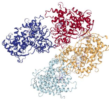
1-rasm. Oqsilning izlangan bo'shliqlarida asetilasetoanilid atsetilgidrazonining o'zaro ta'siri.
