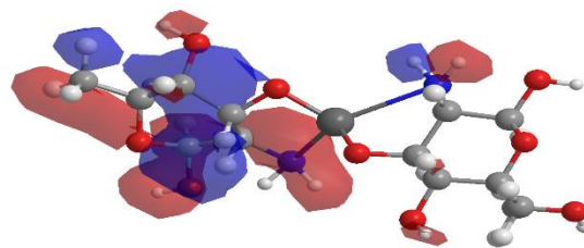
LUMO+49 (N=126) [150,813 eV]
