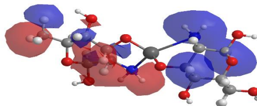
LUMO+49 (N=126) [150,813 eV]
