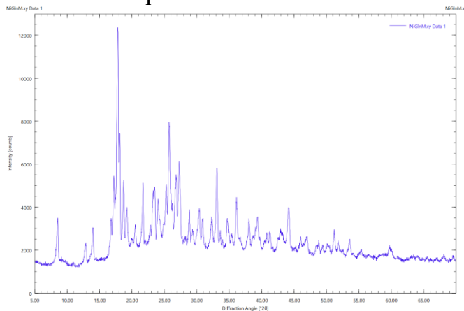
1-rasm. NiGlnAA kompleksi rentgenogrammasi
