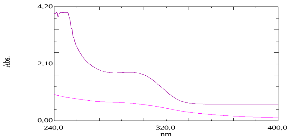
1-rasm. Apis Mellifera xitozani va xitozan- \text{Cu}^{2+} kompleksi UB-spektrlari
