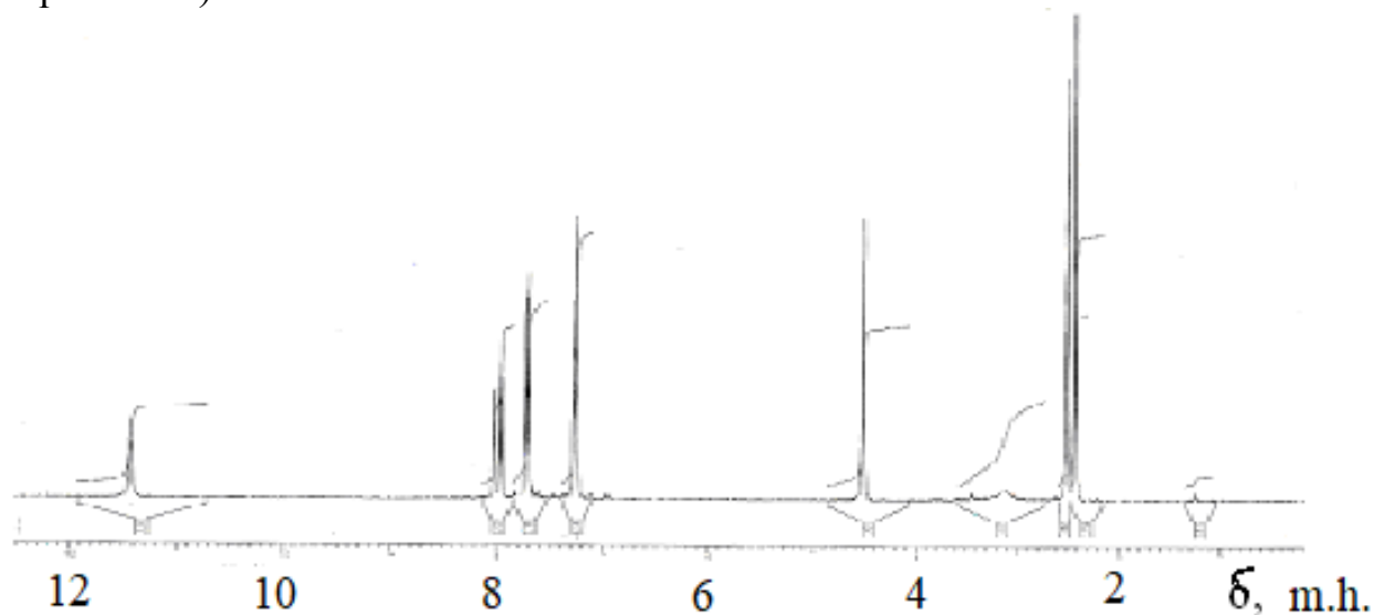
Рисунок 2. ЯМР ^1\text{H} – спектр бензоилгидразона 1-(3-фурила)-4,4,4-трифторбутандиона-1,3 ( \text{H}_2\text{L}^1 ) в растворе \text{DMSO-d}^6
