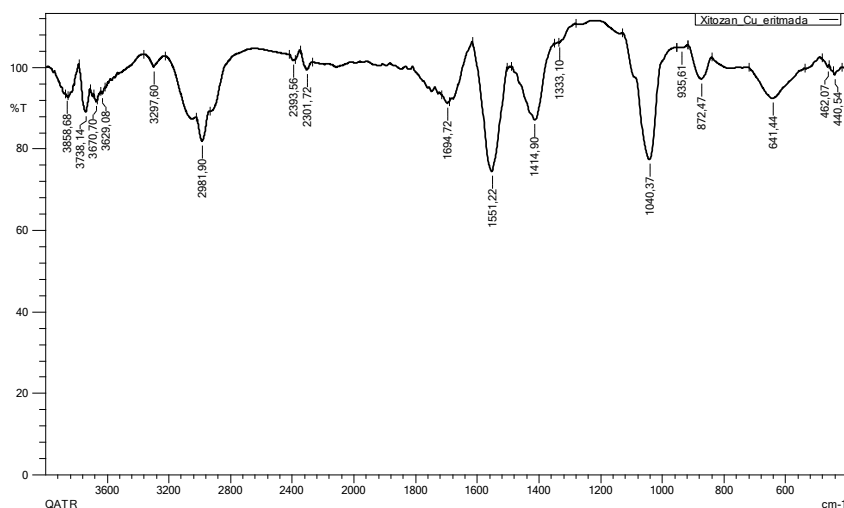
2-rasm. Apis Mellifera xitozaning \text{Cu}^{2+} metalli bilan kompleksi IQ-spektri
