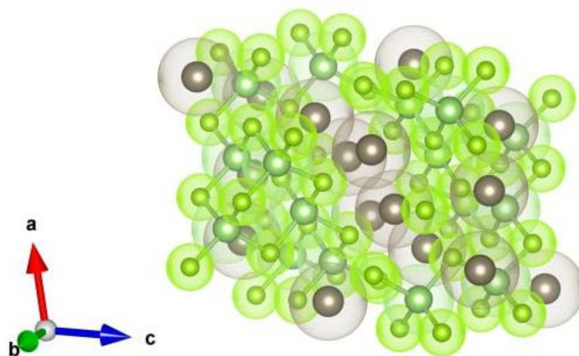
Рис.2. Гексагональная кристаллическая структура \text{TlGaSe}_2 (пр.гр. P6_3/mmc )
