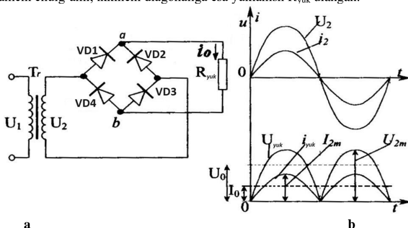
3 – rasm. Ikkita yarim davrli diodli-ko'priksimon to'g'rilagichi: a) chizma, b) tok va kuchlanishlarning grafiklari.
