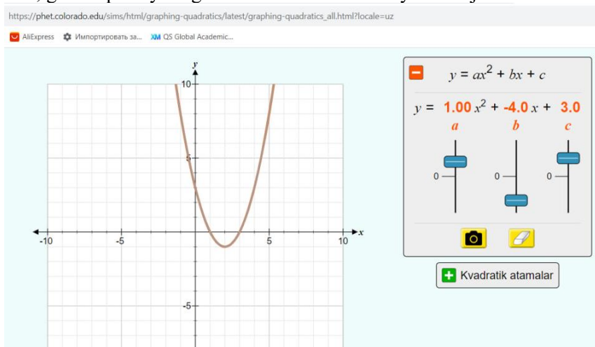
1-rasm. y = x^2 - 4x + 3 funksiya grafigini dastur yordamidagi shakli
