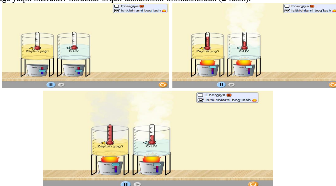
2-rasm. Suyuqliklarni temperatura va ichki energiyasi
