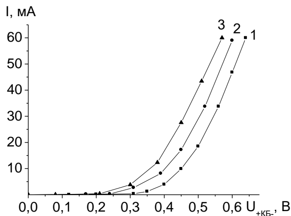
Рис. 1. Зависимости тока от напряжения в режиме прямого смещения перехода коллектор-база при различных температурах:
