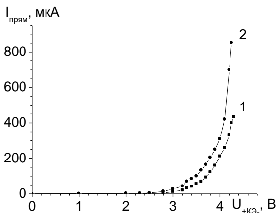
Рис. 3. Зависимости тока от напряжения в двухполюсном режиме включения (+)р-п-р + (-) с плавающей (свободной) базой при запирании эмиттерного перехода: 1 –30°С, 2 –50°С.
