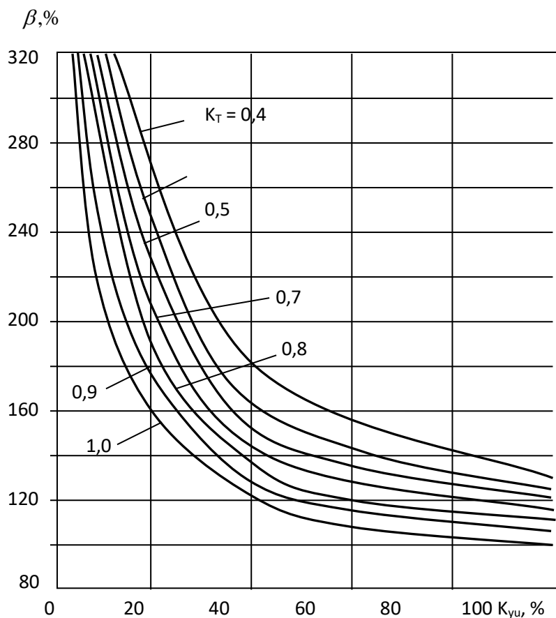
2 – rasm. Ishchi mashinada sarflanayotgan elektr energiya solishtirma qiymatining yuklanish koeffitsiyentiga bog`liqlik grafigi
