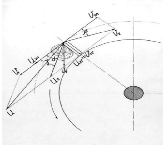
Расм. 3. Пахта чигитининг бўлакчасининг қозикқа урилгандан кейинги абсолют тезлигининг катталиги ва йналиши схемаси.
