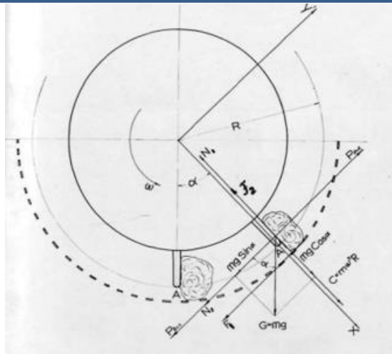
Расм. 4. Чигит саралагич ишчи зонасида пахта чигитига таъсир қилувчи кучлар схемаси.
