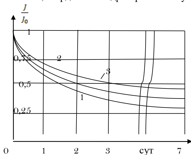
Рисунок 1. Изменение относительной интенсивности аналитических пиков \text{Ca}(\text{OH})_2 в процессе тепло влажностной обработки смесей активная добавка – известь.
