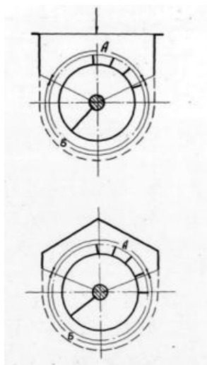
Расм. 2. Чигит саралагич ишчи камерасининг кўндаланг кесими: А-узатиш ва ташлаш зонаси; Б-ишчи зона.
