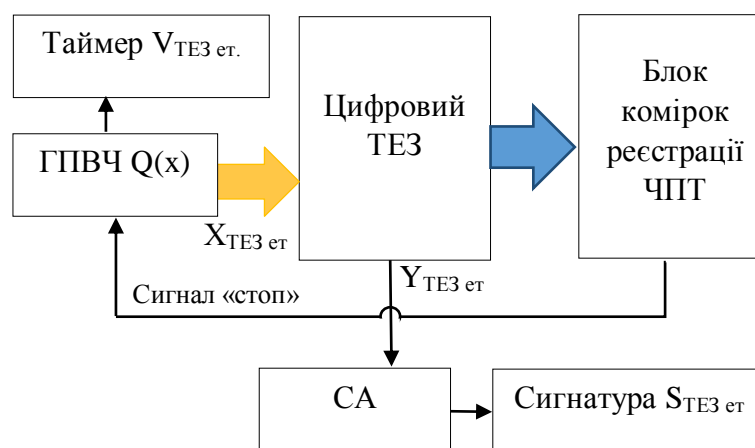
Рис.1 Структурна схема пристрою будови тестової послідовності
