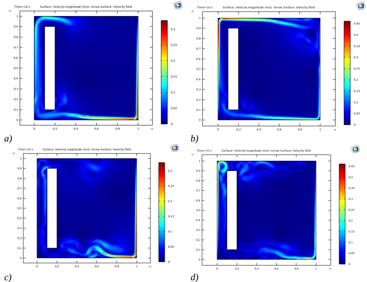
2-rasm. Tadqiqot ob'yektida havo tezligining o'zgarishi: a - boshlang'ich vaqtda; b - 16 s dagi holat; c - 25 s dagi holat; d - 100 s dagi holat.
