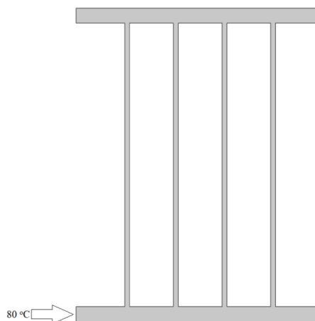
Рис. 5. Общий вид радиатора.
