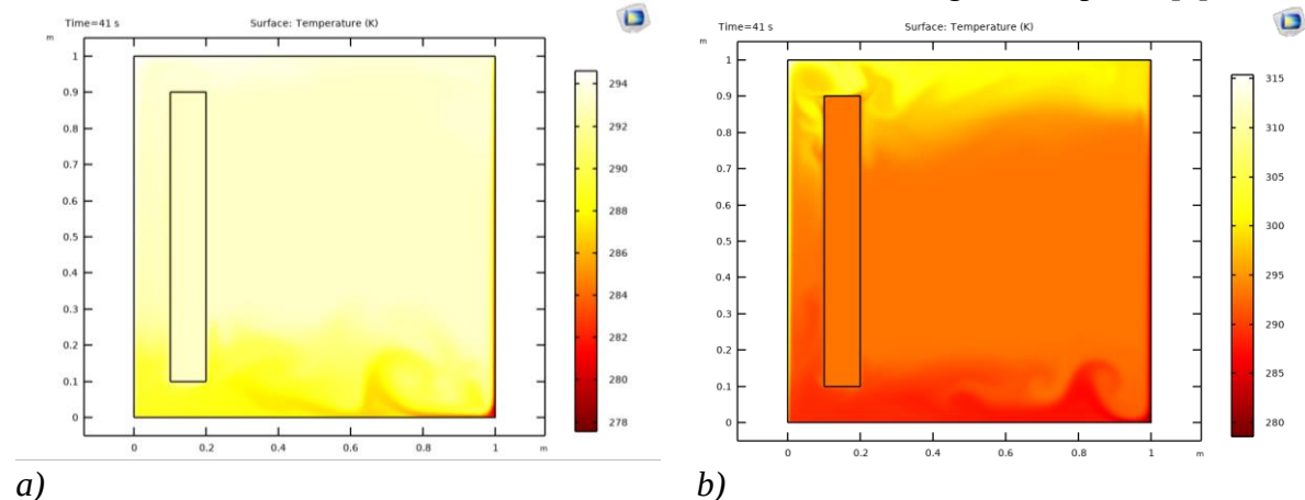
3-rasm. Tadqiqot ob'yektida temperatura taqsimoti: a - 41 s dagi holat; b - 100 s dagi holat.
