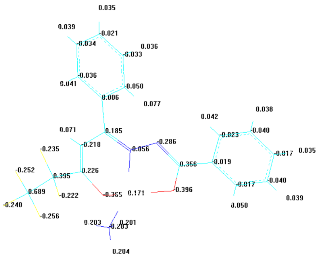
1-rasm. NiL^7 \cdot NH_3 kompleks birikmasi tarkibidagi atomlar o'rtasidagi bog'larning effektiv zaryadlari
