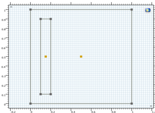
1-rasm. Tadqiqot ob'yektining Comsol Multiphysicsda geometrik ko'rinishi.
