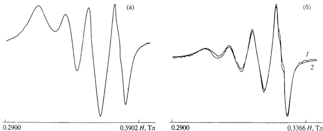
2-расм. Мис (II) нинг гомобиядроли комплекси Cu_2L^1 \cdot 2NH_3 [Cu(II) – Cu(II)] – (а) ва гетеробиядроли комплекси NiCuL^1 \cdot 2NH_3 [Ni(II) – Cu(II)] – (б) толуол+хлороформдаги эритмаларининг ЭПР спектрлари (1 –экспериментал спектр, 2 – назарий ҳисоблаб топилган спектр)
