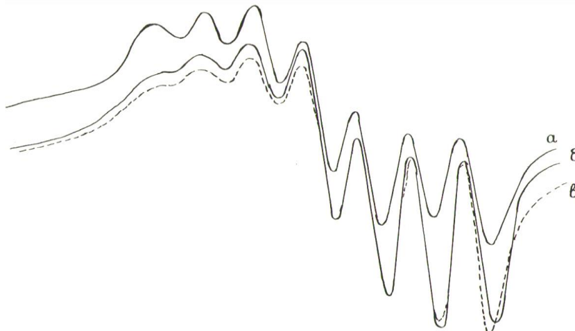
1-расм. Мис(II) биядроли комплексларининг ЭПР спектрлари: Cu_2L^1 \cdot 2NH_3 – (α) ва Cu_2L^2 \cdot 2NH_3 – (β) толуол эритмасида 300 К да; назарий – (γ)
