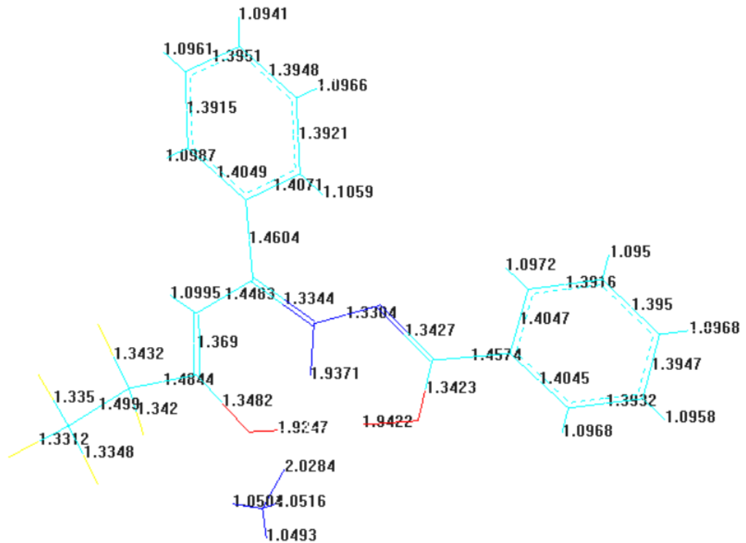
2-rasm. \text{NiL}^7 \cdot \text{NH}_3 kompleks birikmasining atomlar o'rtasidagi bog' uzunligi Hyperchem dasturi hisoblashlariga ko'ra, kompleks tarkibidagi eng muhim geometriya elementlari quyidagicha bo'ldi:
