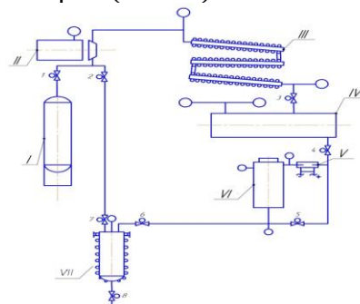
2-rasm. Tajriba qurilmasining prinsipl sxemasi.
