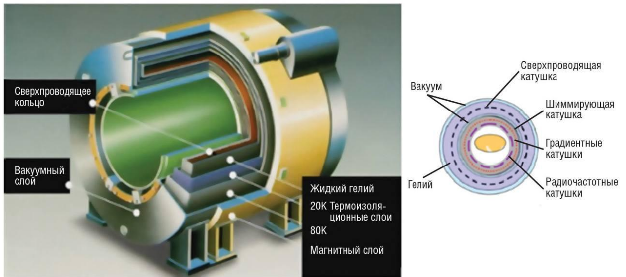
4-rasm. MRT apparatida O'ta o'tkazuvchi magnitning tuzilishi.
