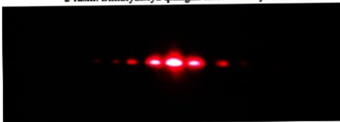
3-rasm: Haqiqiy interferentsiya sxemasi
