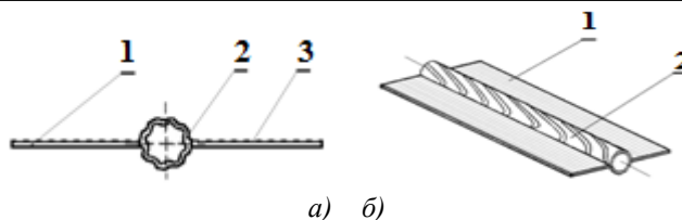
а) б) Рис.1 – Плоская теплоприемная панель гелиоколлектора с витым теплоотводящим каналом (а), общий вид теплоприемной панели (б).
