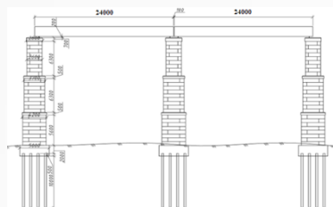
1-расм. Тошкент – Самарқанд тезликли автйўл трассаси автйўл эстакадасининг I-варианти
