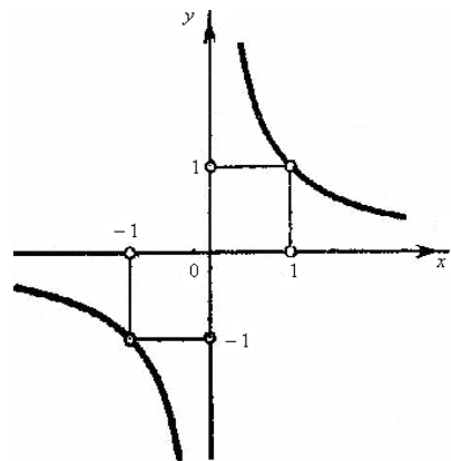
y = \frac{1}{x} giperbola.
