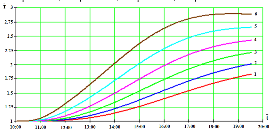
Рис.4. Изменения безразмерной температуры по слоям дыни по времени. 1- при \bar{x} = 0,3 , 2- при \bar{x} = 0,4 3- при \bar{x} = 0,5 4- при \bar{x} = 0,6 , 5- при \bar{x} = 0,7 , 6- при \bar{x} = 0,8
