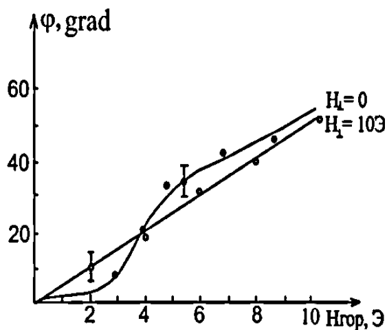
Рис.3. Изменение поворота ПДС в зависимости от приложенного внешнего поля.
