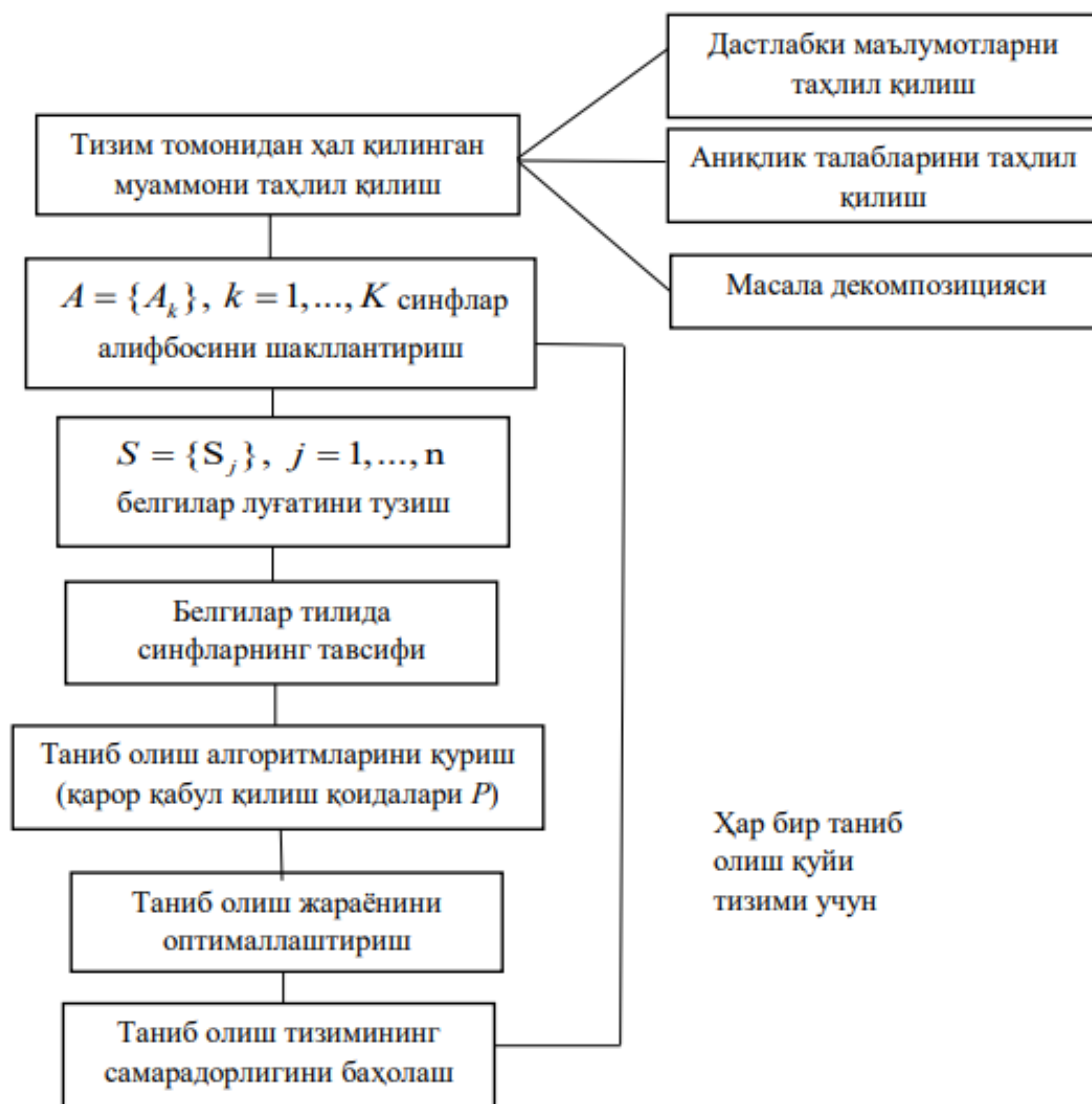
1- расм. Таниб олиш тизимини қуришнинг умумий схемаси.
