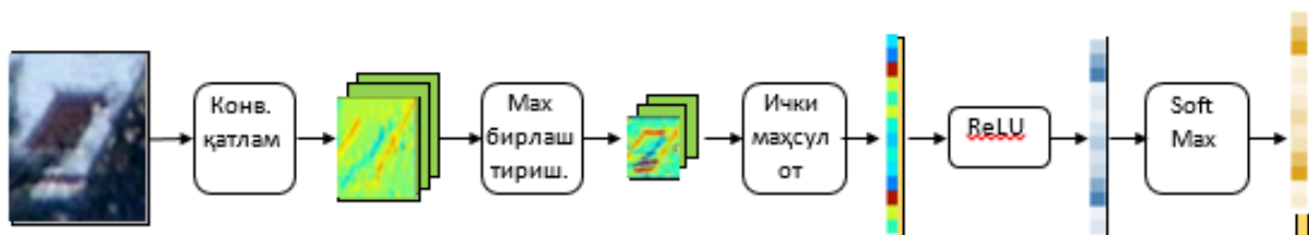
1-расм. Одатда энг кўп ишлатиладиган қатламлардан ташкил топган оддий CNN архитектураси.
