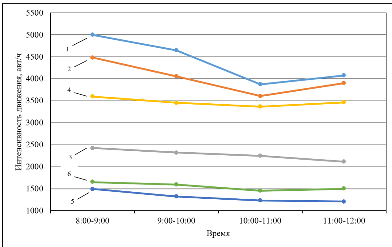
Рис. 1. Интенсивность движения на объекте исследования:
