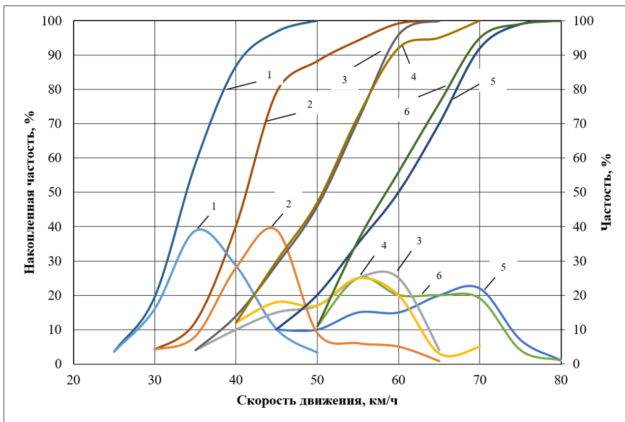
Рис. 3. Модальные и кумулятивные кривые скорости движения:
