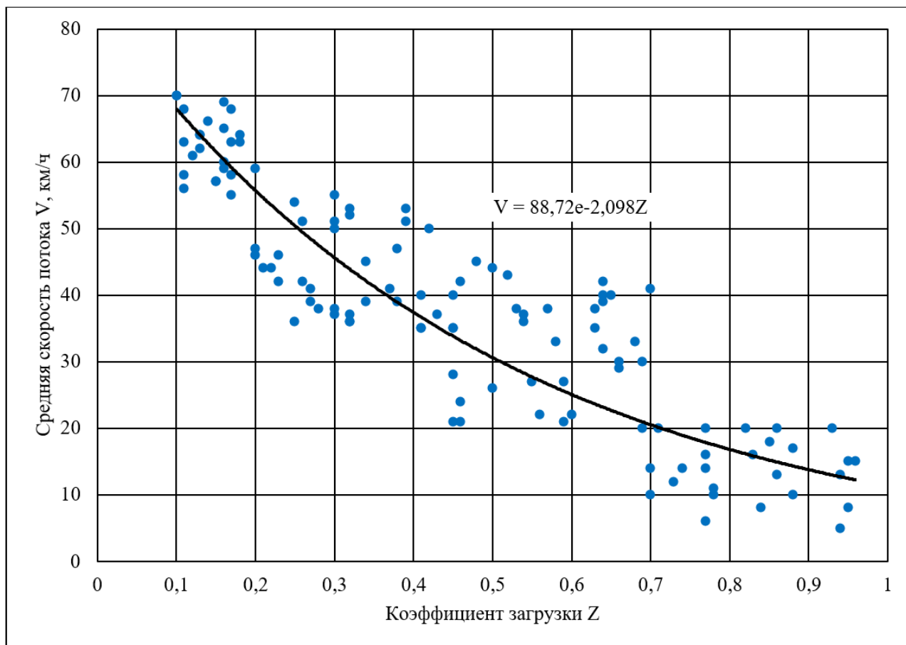
Рис. 4. График закономерности между скоростью и уровнем загрузки движения при различных условиях движения.
