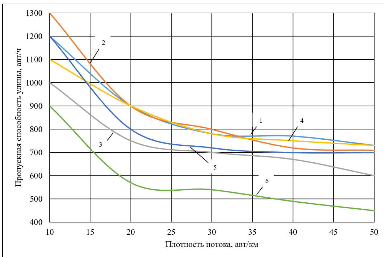
Рис. 5. График зависимости между плотностью потока и пропускной способностью улицы:
