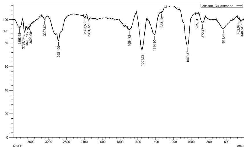
2-rasm. Apis Mellifera xitozaning Cu^{2+} metalli bilan kompleksi IQ-spektri
