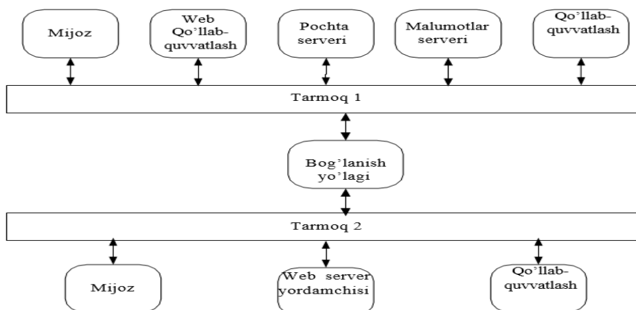
1-rasm. Qo'shma konferensiyani boshqarish tizimining arxitekturasini
