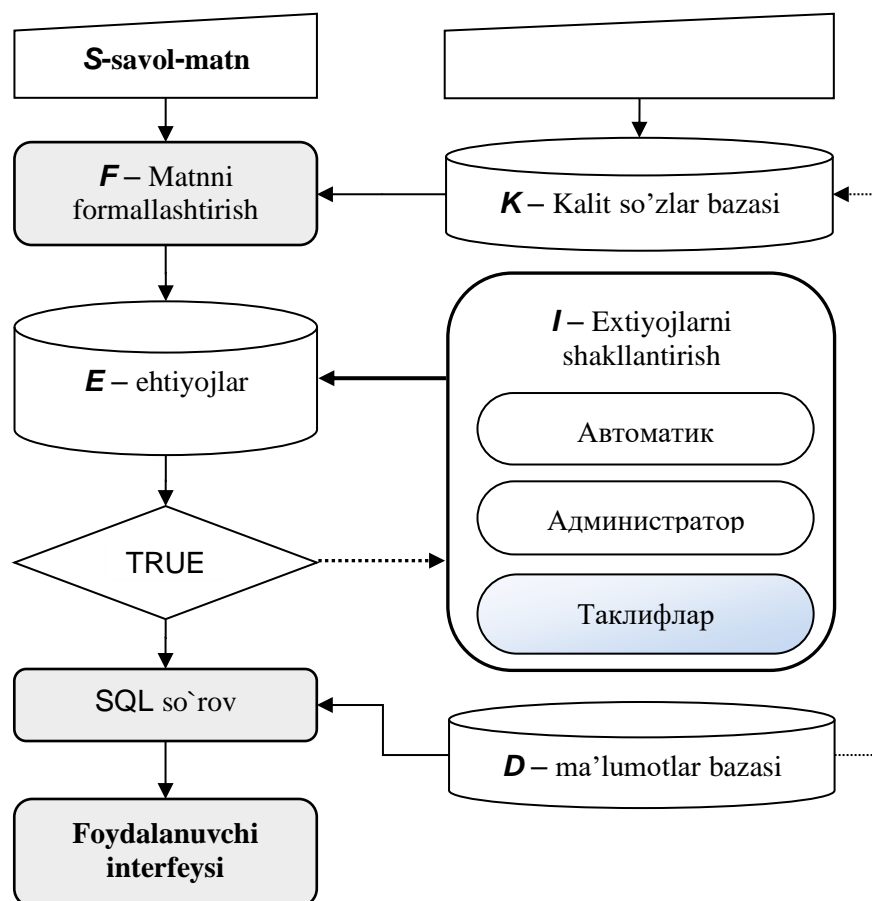
1- rasm. Soliq tushumlarini bashoratlashga ko'maklashuvchi axborot tizimi tuzilmasining SQL translyatsiyasi algoritmi
