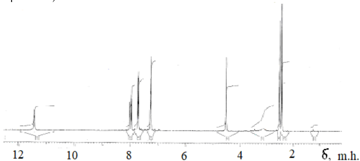
Рисунок 2. ЯМР ^1\text{H} – спектр бензоилгидразона 1-(3-фуранила)-4,4,4-трифторбутандиона-1,3 ( \text{H}_2\text{L}^1 ) в растворе \text{DMSO-d}^6
