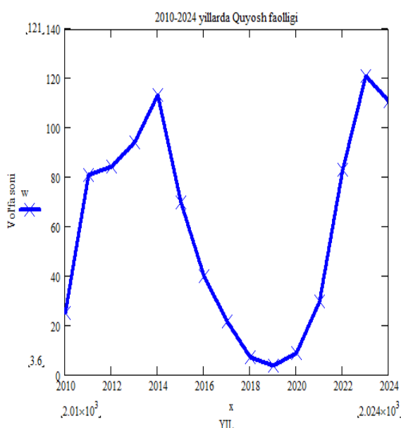
1-chizma. 2010 yildan to 2024 yil aprel oyigacha Quyosh faolligining Vol'fa sonlarida o'zgarish dinamikasi
