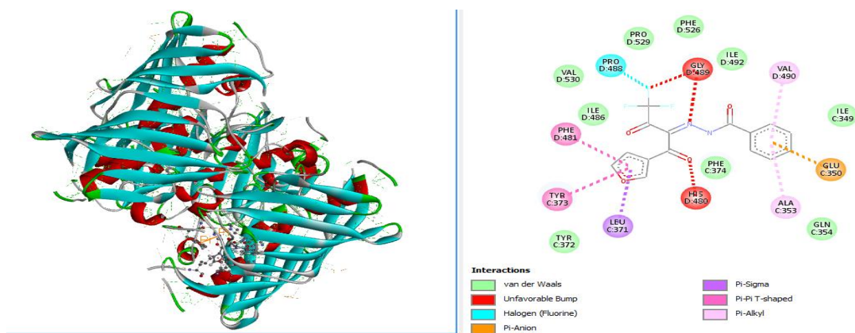
Рис.3. Результаты молекулярного докинга молекулы H_2L^1
