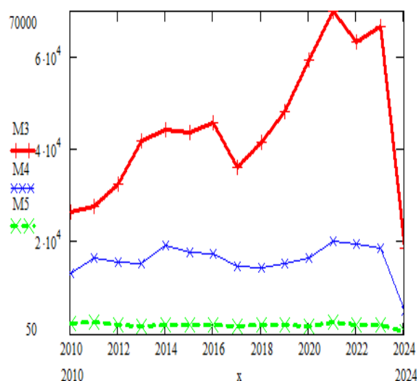
2-chizma. 2010 yildan to 2024 yil aprel oyigacha Yer sharida 3 magnitudadan yuqori (M3), 4 magnitudadan yuqori (M4) va 5 magnitudadan yuqori (M5) Yer qimirlash-lar sonining o'zgarish dinamikasi
