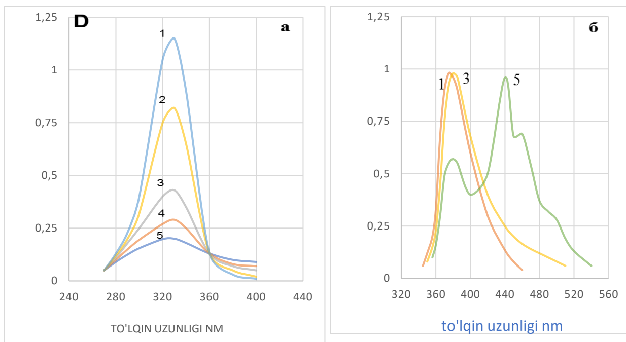
1-rasm. Doimiy dioksan-suv ikkilik aralashmasidagi 1-1-(4-tolil)-2-(4-bifenil)etilenning yutilish (a) va floresans (b) spektrlarining konsentratsiyaga bog'liqligi 1:10^{-5} (1), 4,10^{-5} (2), 10^{-4} (3), 2,10^{-4} (4), 5,10^{-4} M (5)
