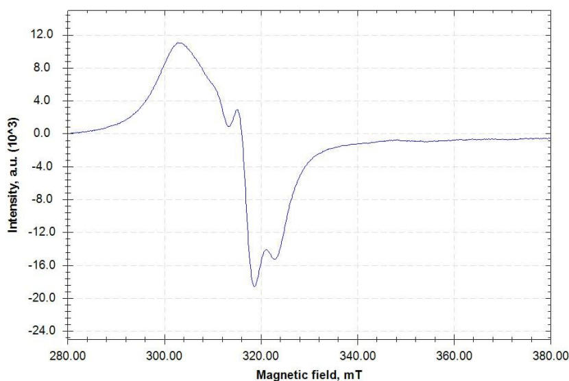
3-rasm. Apis Mellifera xitozaning Cu^{2+} metalli bilan kompleksi EPR-spektri
