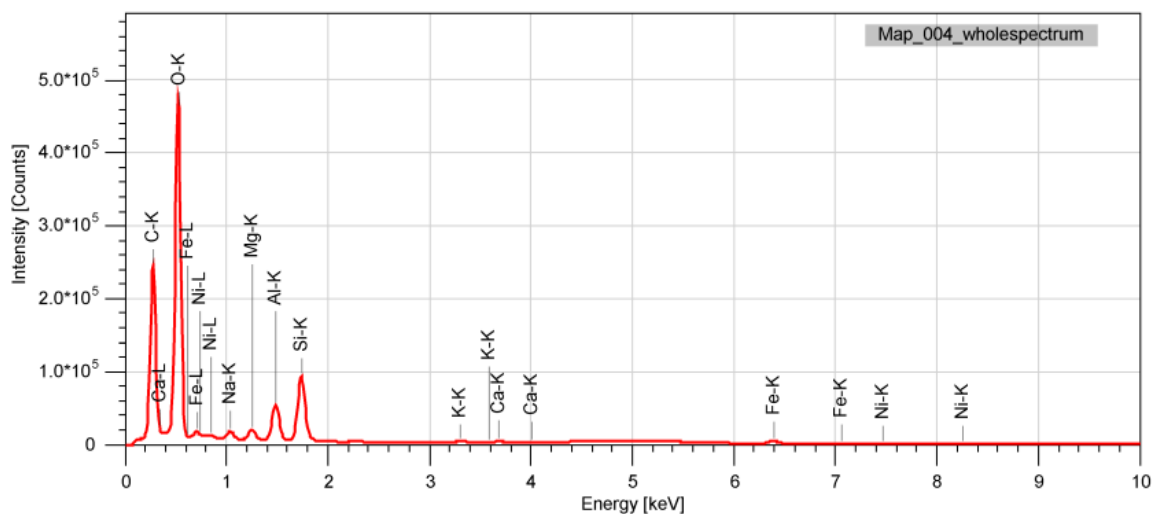
3-rasm. Kimyoviy tahlillar uchun tanlab olingan 7-shisha namunasining Skanerlovchi elektron mikroskop (SEM-EDS) da olingan spektrlari
