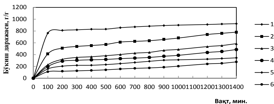
1- расм. Бентонитнинг турли масса улушида полимер композицияларнинг t= 25^{\circ}\text{C} да дистилланган сувдаги бўкишининг кинетик эгри чизиқлари:
