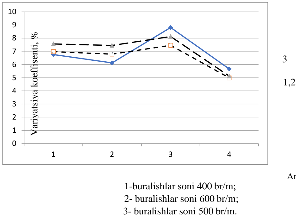
3.5-rasm. Paxta va ikkilamch tolalar aralashmasidan olingan iplarning uzilish kuchi bo'yicha variatsiya koeffisientining o'zgarishi.
