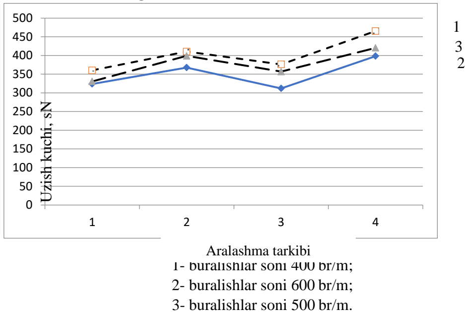
3.3-rasm. Paxta va ikkilamch tolalar aralashmasidan olingan iplarning uzilish kuchining o'zgarishi.
