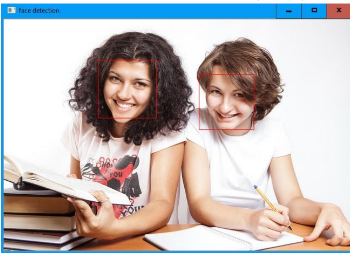
Рис.3.7. Тестирование программы
