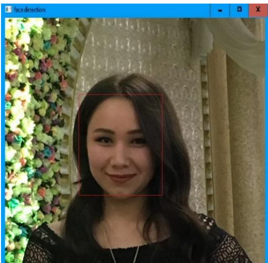
Рис.3.7. Тестирование программы
