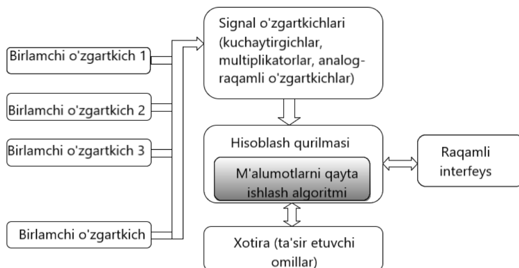
1-rasm. Intellektual datchikning struktura sxemasi.
