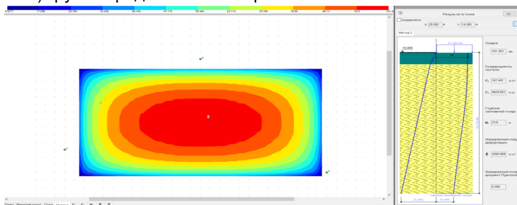
Рис.4. Результаты расчета фундамента и грунта
