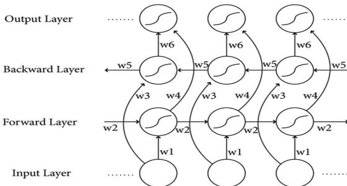
4-rasm BiLSTM tarmoq strukturasi diagrammasi
