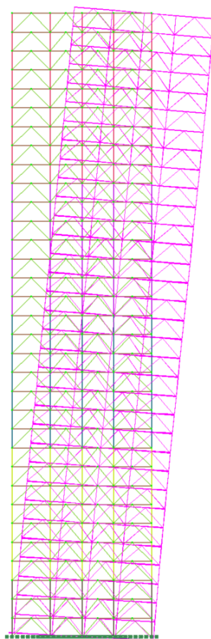
Рис. 5. Деформированная схема каркаса от сейсмической нагрузки
