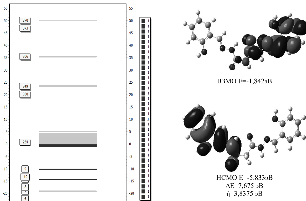
Рисунок 1. Диаграмма энергетических уровней МО (ВЗМО-НСМО) N 1 ,N 3 -бис-((E)-2-гидроксibenзилиден) малоноилгидразона
