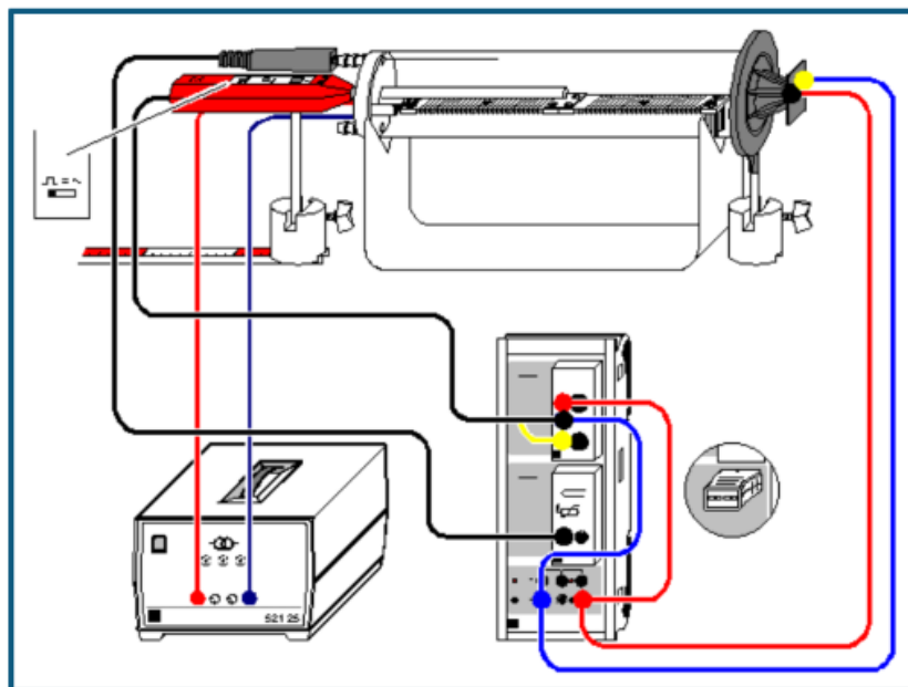
2- rasm. Tovushning havodagi tezligini aniqlash qurilmasi sxemasi
