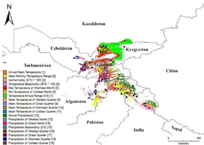
6-расм. R. rubrocalyx гербарий намуналари мавжуд координаталарга чекловчи биоиклимий тенденциялар таъсири
