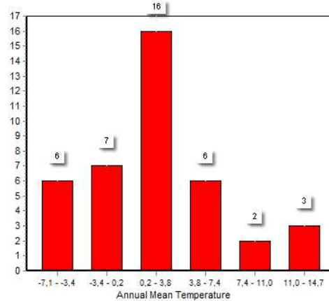
2-диаграмма. R. rubrocalyx гербарий намуналари мавжуд координаталарнинг йиллик ўртача ҳарорат бўйича тақсимланиши
