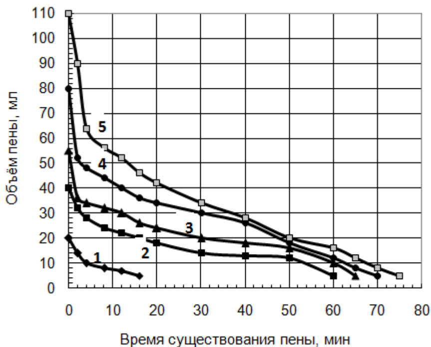
Рис. 2. Кинетика разрушения пны при различной концентрации МДТМ в собирательной смеси МДТМ:СМ при соотношении 3:1 1 – 0,24 %; 2 – 0,32 %; 3 – 0,4 %; 4 – 0,48 %; 5 – 0,56 %
