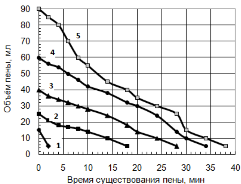
Рис. 4. Кинетика разрушения пены при различной концентрации МДТМ в собирательной смеси МДТМ:СМ при соотношении 1:1
