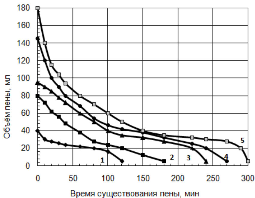
Рис. 1. Кинетика разрушения пены при различной концентрации МДТМ:
