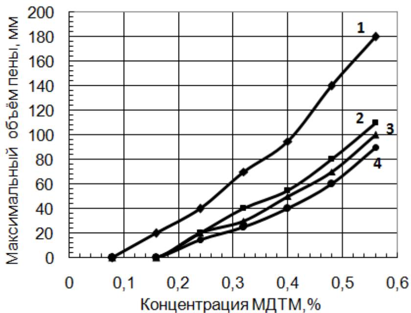
Рис. 5. Зависимость максимального объёма пены от концентрации МДТМ при различном соотношении МДТМ:СМ в собирательной смеси:
