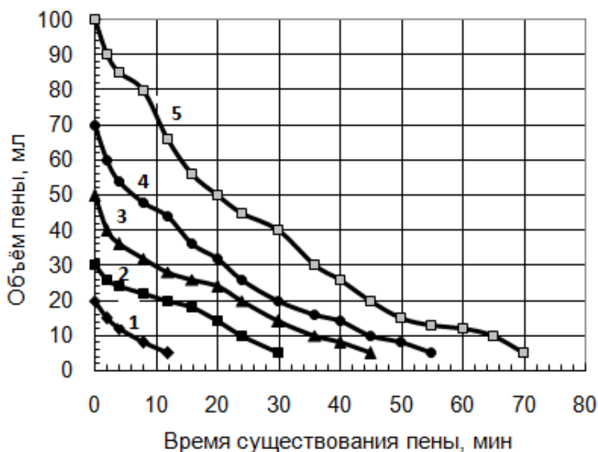
Рис. 2. Кинетика разрушения пны при различной концентрации МДТМ в собирательной смеси МДТМ:СМ при соотношении 3:1 1 – 0,24 %; 2 – 0,32 %; 3 – 0,4 %; 4 – 0,48 %; 5 – 0,56 %
