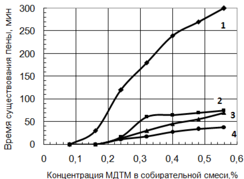
Рис. 6. Зависимость времени существования пены от концентрации МДТМ при различном соотношении МДТМ:СМ в собирательной смеси
